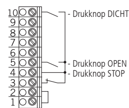
Drukknop OPEN/STOP/DICT (4-aderige oplossing)
