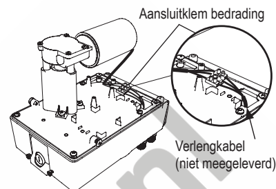
Afbeelding 7 Secundaire eenheid
