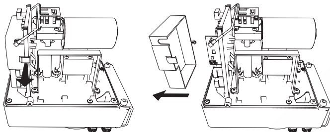
Afbeelding 6 Primaire eenheid
