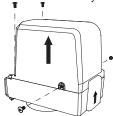
Rys. 5 Zdejmowanie obudowy
