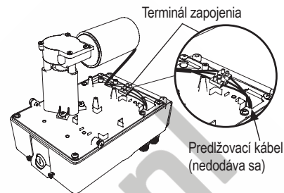
Obrázok 7 Sekundárna jednotka
