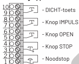
Bedieningsapparaten
