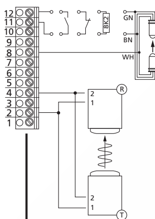
Ingang 2 (11 + 12) Doorgangsfotocel (2 + 4)
