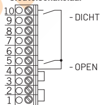
Sleutelschakelaar
