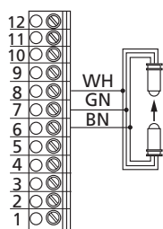
Sluitkantbeveiliging OSE
